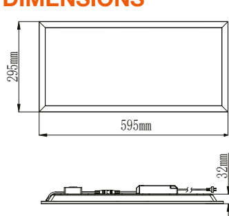
20/15W 595x295x32mm
