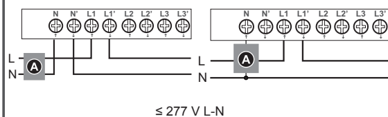
1PH2W LN
