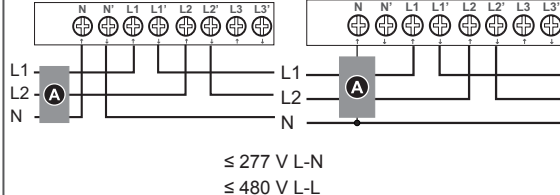
1PH3W LLN
