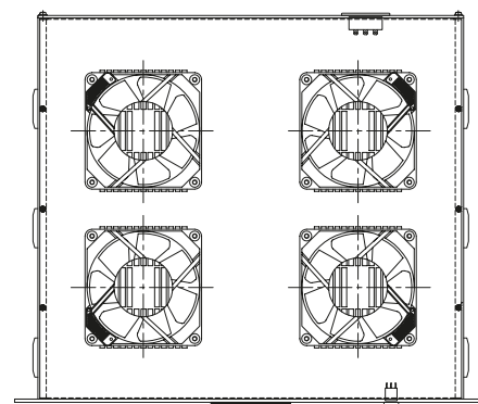
Fan unit top mount
