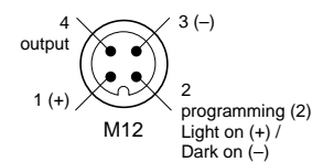
NPN
