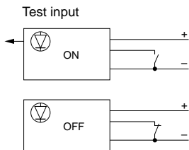
NPN
