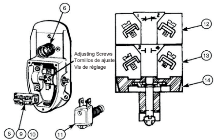
Figure / Figura / Figure 2 : Foot Switches / Interruptores de pedal / Interrupteurs à pédale
