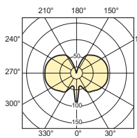
CDM-T Elite 70W /930, /942
