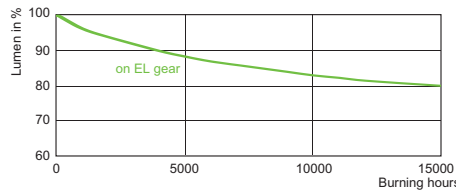
CDM-T Elite 35W & 70W /930
