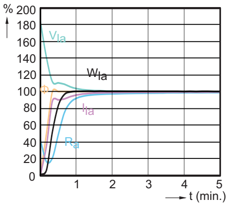
CDM-T Elite 50W /930
