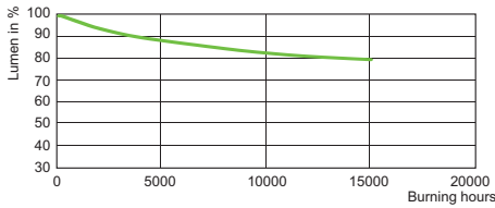
CDM-T Elite 50W /930
