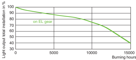
CDM-T Elite 70W /930
