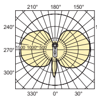
CDM-T ELITE 150W
