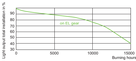
CDM-T Elite 50W, 70W /942
