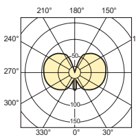
CDM-T Elite 35W /842, /930, /942
