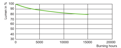
CDM-TC Elite 50W /930
