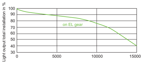
CDM-T Elite 50W, 70W /942
