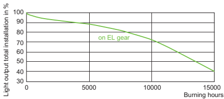
CDM-T Elite 35W /842, /942
