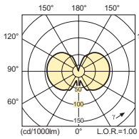
CDM-TC Elite 50W /942
