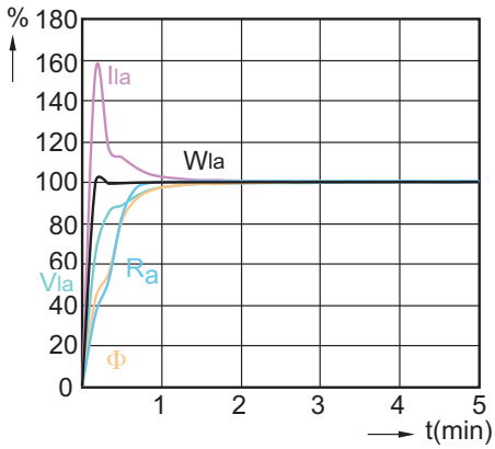
CDM-TC Elite 50W /942
