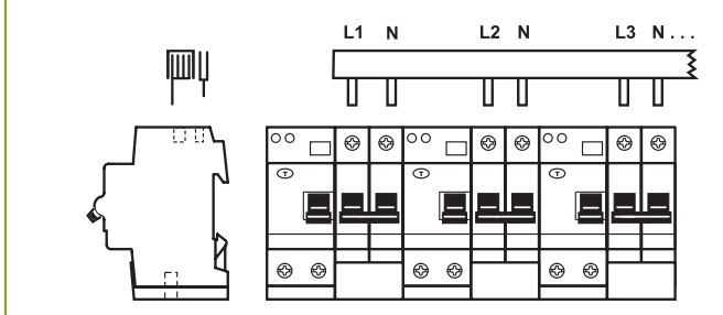
PS 4/30/16N-DDA 202 T DS 202 + DS 202 + (DDA 202 + S 202) ...
